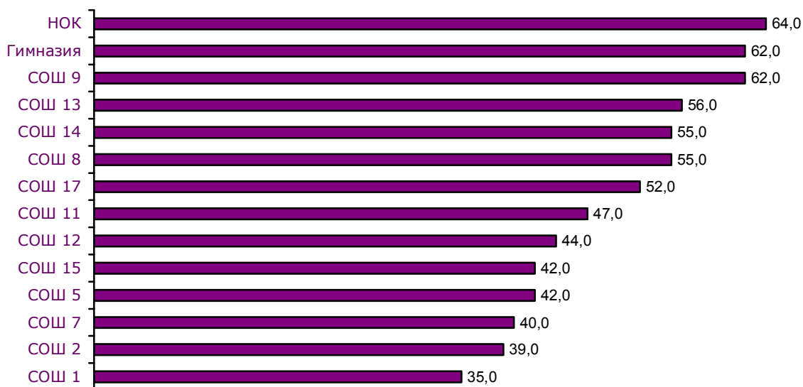
Рисунок 3. Средние баллы ЕГЭ по предмету «Математика» (профильный уровень)
